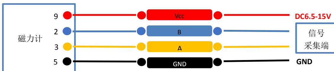
图 5-1-2 RS485 接口接线图
