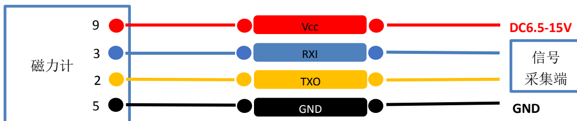
图 5-1-1 RS232 接口接线图
